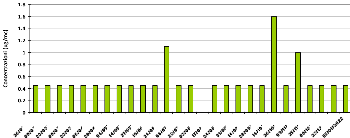
Sito 08 - Diagramma dei valori di concentrazione di H2S rilevati.
