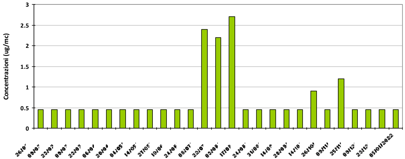
Sito 12 - Diagramma dei valori di concentrazione di H2S rilevati.
