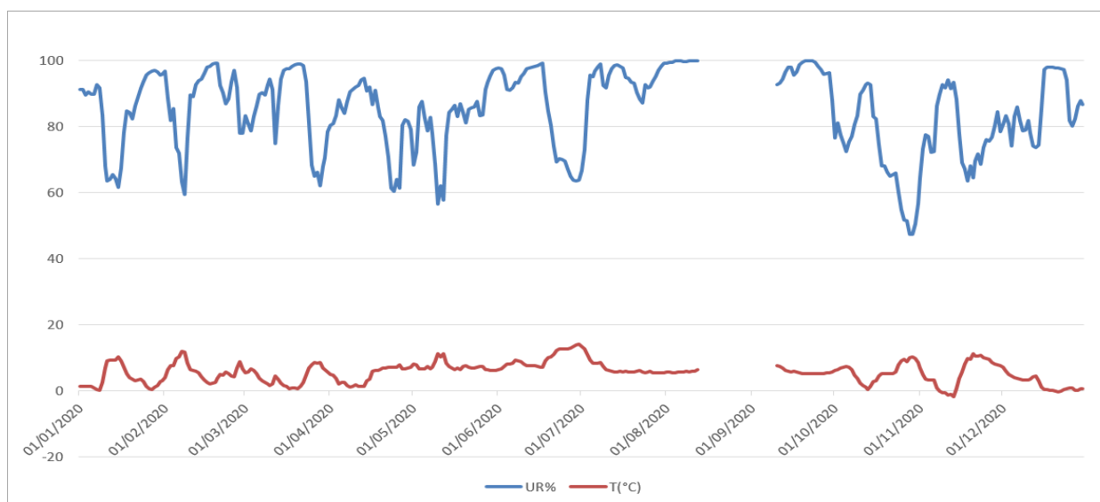
Figura 7.1 - Andamento dell'Umidità relativa (UR) e della Temperatura nel periodo di riferimento – Stazione di Viggiano
